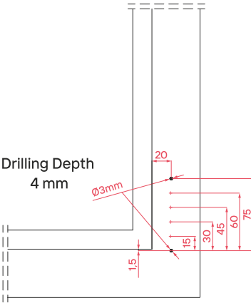
Frame Hinge Bottom
